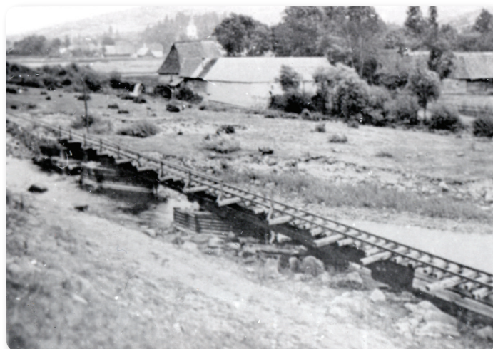
Železničný most cez potok Studená pri obci Biely Potok © reproto publikácie Oravský komposesorát, Praha 1930
